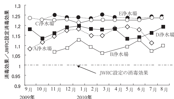
図16 各浄水の消毒効果の推定値 (JWRC技術審査基準との比較)
