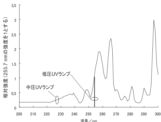
図14 中圧および低圧UVランプの照射スペクトル (254nmの照射強度を1とした場合の相対値)
