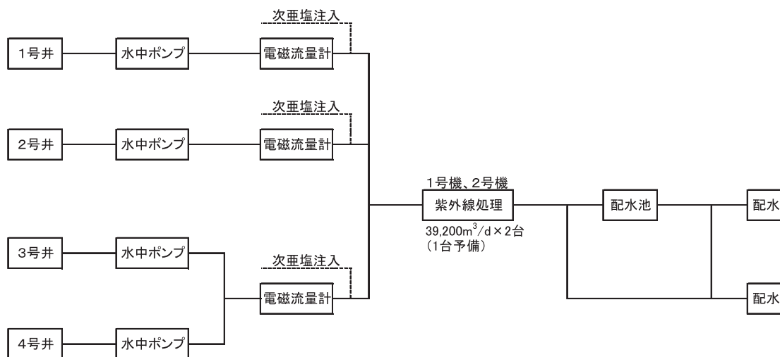
紫外線処理関連フロー
